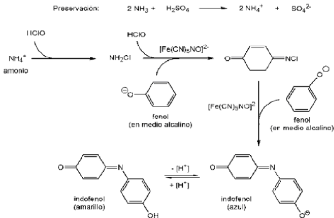
Fig. B.7.4-1. Formación del indofenol de color azul producto de la reacción del ión amonio con hipoclorito y fenol en medio básico en presencia de nitroferriicianuro.
